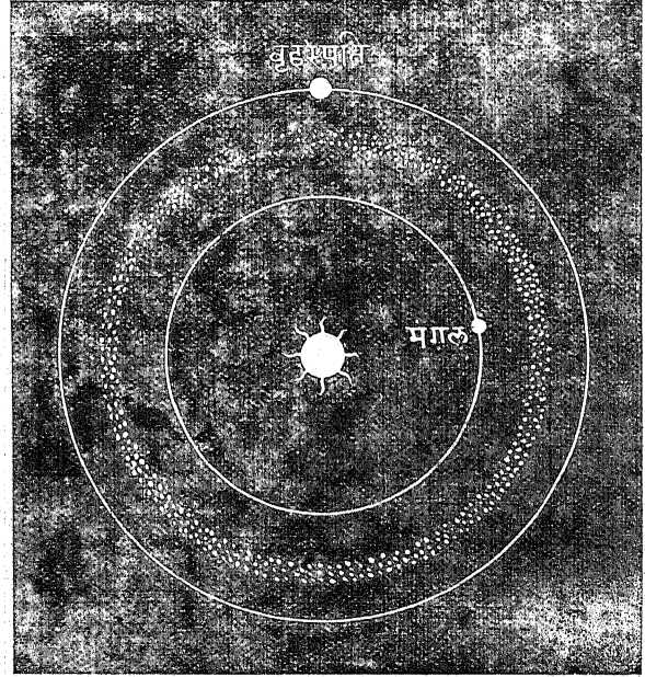
चित्र ३३—मंगल और गुरु के बीच असंख्य
